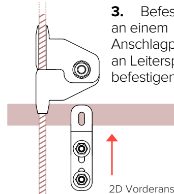
2D Vorderansicht
