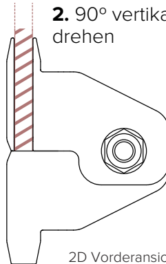
2D Vorderansicht
