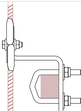
2D Vorderansicht
